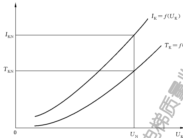
图 3 堵转特性曲线
